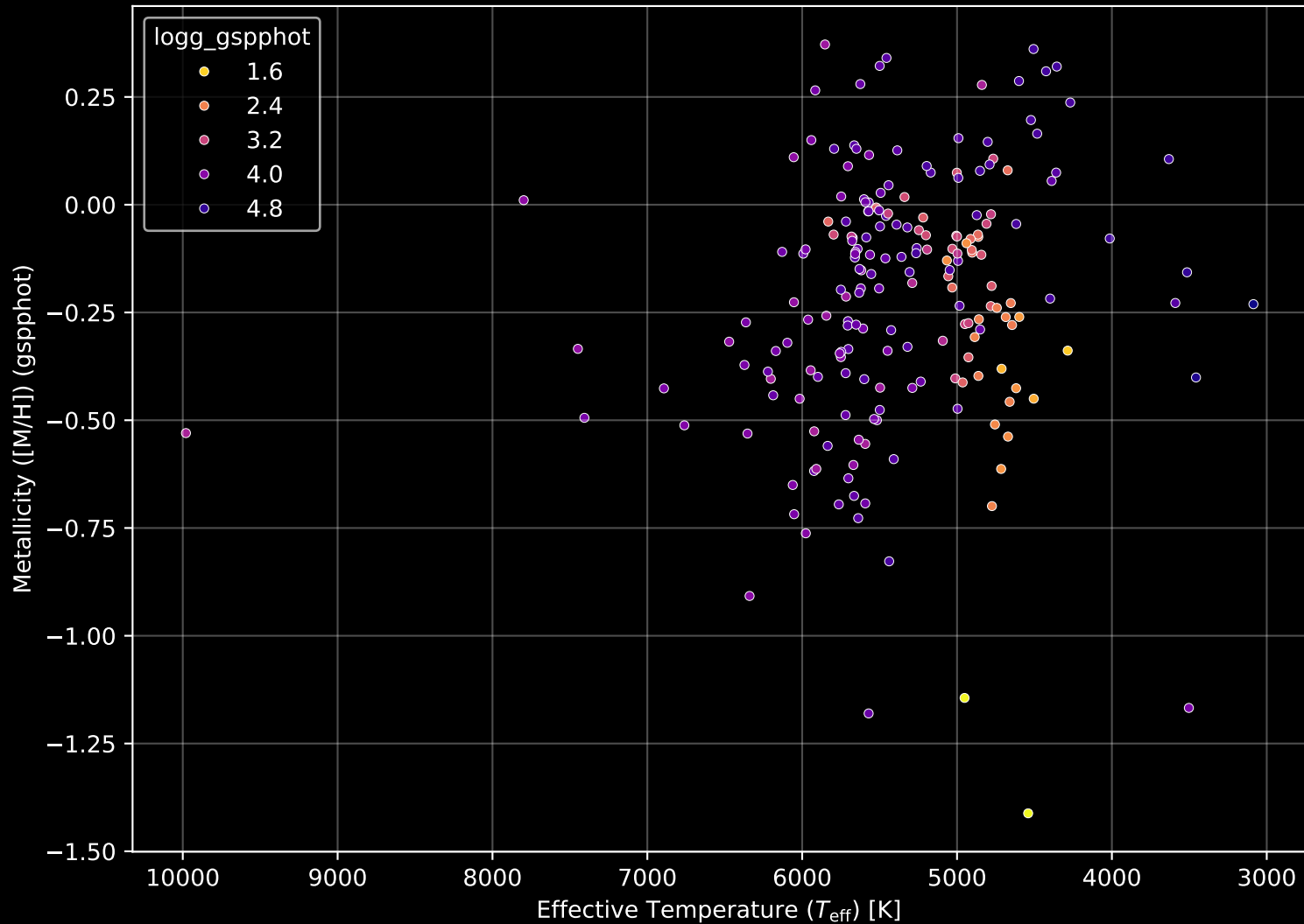
APOGEE DR17 Field: [267-32-O_TESS] Stellar Population Parameters (n= 200)
